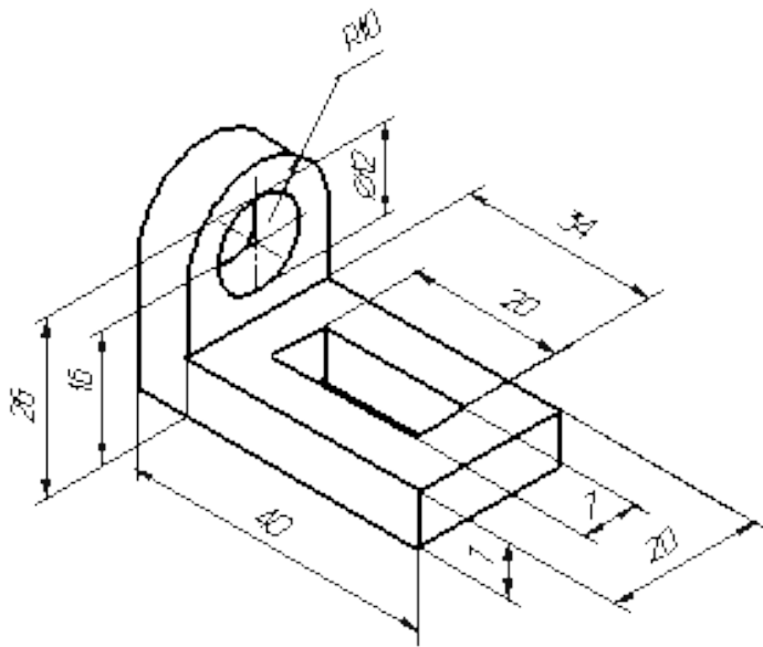
Рис. 1. Кронштейн
